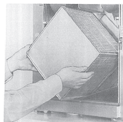
Dra ut värmeväxlaren.
