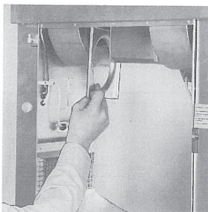
Lossa vingmuttern och ta bort inloppsramen.
